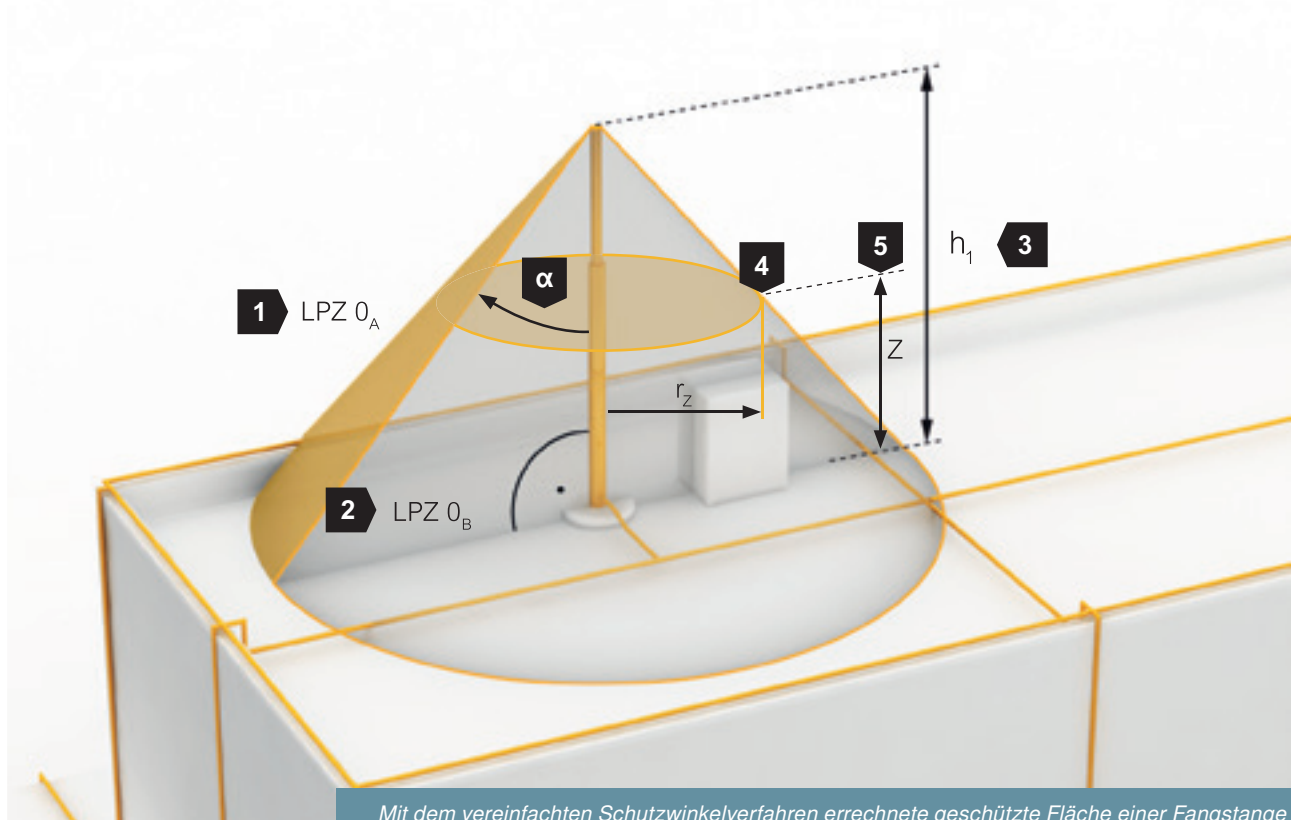
Schutzwinkel nach Blitzschutzklasse nach VDE 0185-305-3 (IEC 62305-3) für Fangstangen bis zu 2 Metern Länge
